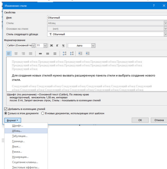
Рисунок 2 - Изменение стиля
