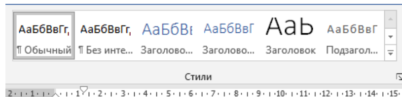
Рисунок 1 - Стили
