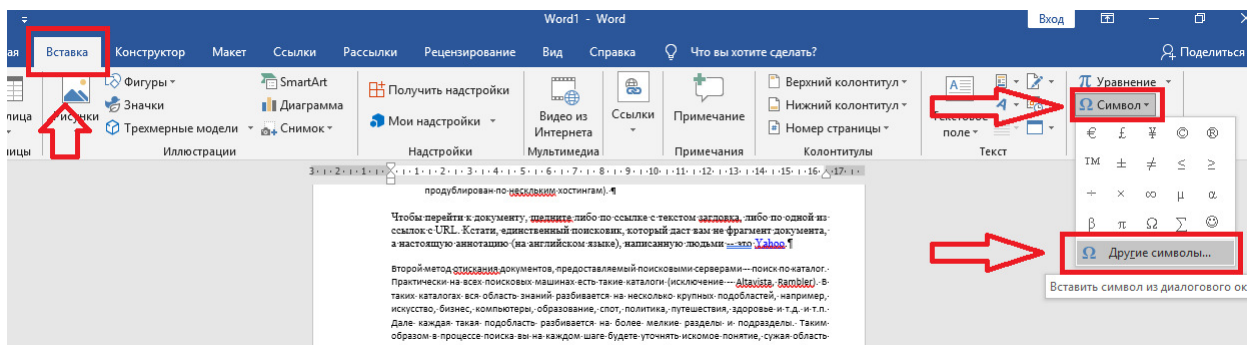
Рисунок 5 - Ввод символов
