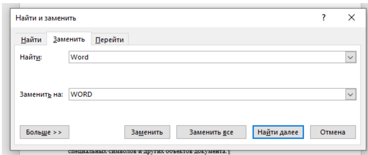
Рисунок 3 - Замена текста
